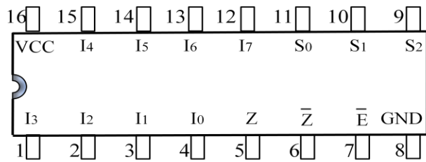
74xx151
